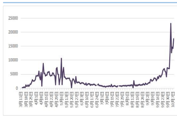
图：英国 日新增病例趋势
