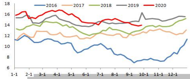
钢厂焦炭库存可用天数
