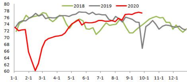
焦炉产能利用率 (230家)
