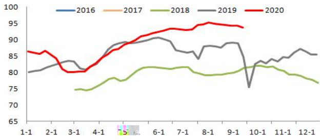
高炉产能利用率
