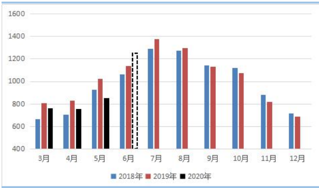
1: 水力发电产量 单位: 亿千瓦时
